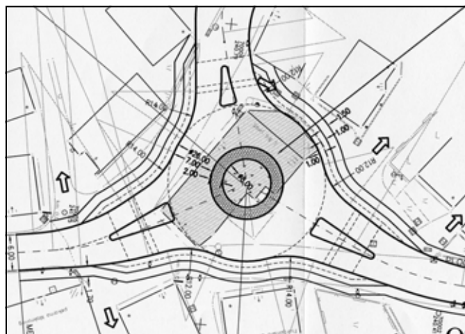
Slika 2: Ureditev križišča v obliki krožnega križišča, izsek iz idejnega projekta (IDZ št. 1357) ureditve križišča v Mokronogu na R!-215, odsek 1163 Trebnje-Mokronog-Boštanj, km 0.000. Izdelovalec: Projektivni biro Lunar d.o.o. iz Kranja.
